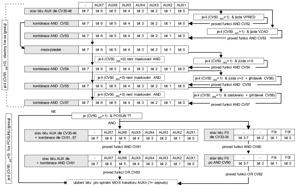
Tab4. zpracování logiky výstupů AUX1-AUX7 dle CV50-CV57 + režim POSUN
